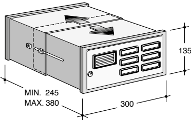
placca per pulsantiera profondità regolabile (senza accessori) plate for push-button panel with adjustable depth (without accessories)
