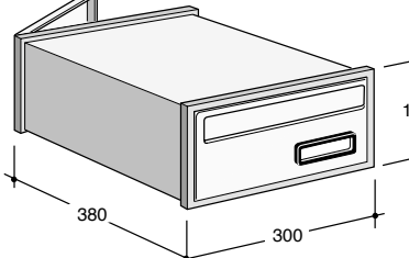
cassetta postale profondità regolabile letterbox with adjustable depth
